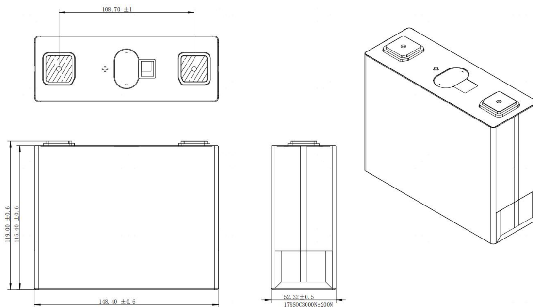
电池尺寸/mm
